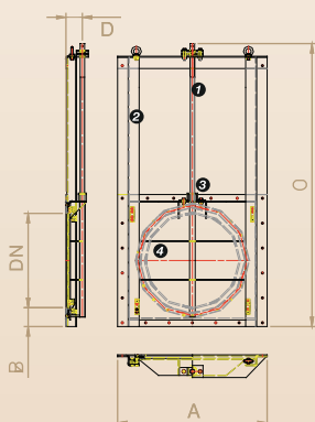
Základní rozměry [mm]
