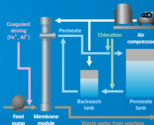
Membrane module installation
